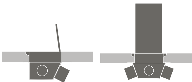
Steckerwanne einseitig und zweiseitig bedienbar power outlet box with hinged lid, one side or both sides useable
